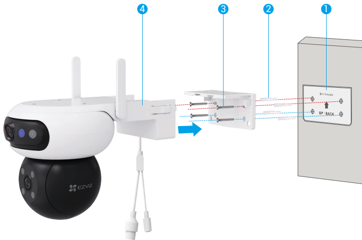
圖 2 壁掛式安裝
